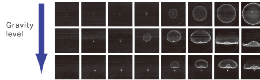
過重力環境下での定容爆燃現象
