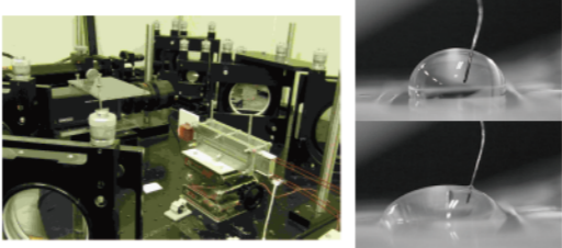
2波長干渉計による多成分ヒートパイプの解析 エレクトロウエッティングによる液滴形状の制御
