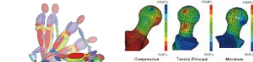
高齢者転倒シミュレーションと骨折リスク評価
