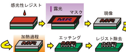
フォトリソグラフィによる微細加工
