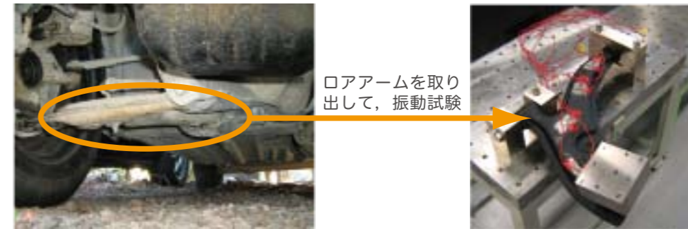
回転自由度を考慮した伝達経路解析の開発と自動車への適用例 (目的: タイヤから車体に伝わる力を知る)
