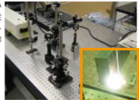
レーザーアブレーションの瞬間
