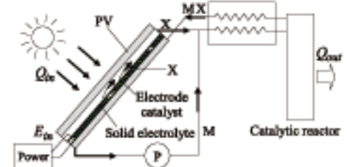
太陽電池冷却・ヒートポンプ熱利用システム
